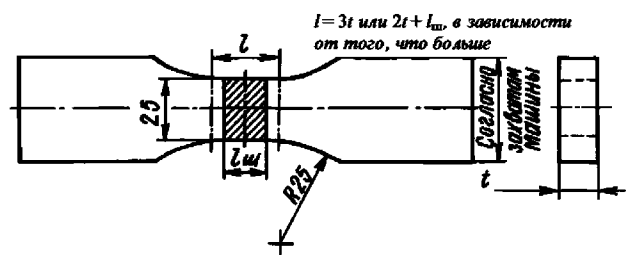
Рис. 4.2.2.1 Поперечный образец для испытаний на статическое растяжение:
