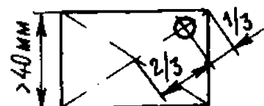
Рис. 3.2.5-5 Пруток прямоугольного сечения
