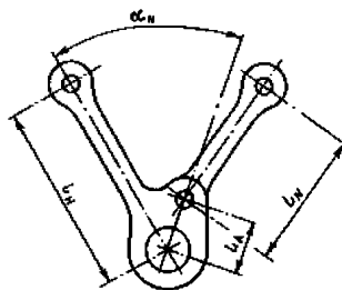
Рис. 2.4.3-2 Прицепной шатун
