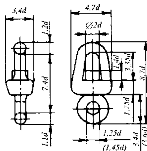
Рис. 7.1.3-7 Вертулюг
