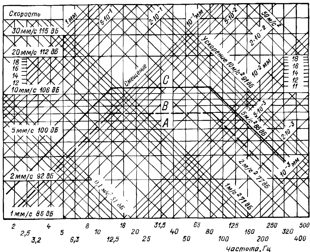
Рис. 9.5.4 Нормы вибрации генераторов ДЦ, валогенераторов, турбоприводов и турбогенераторов мощностью 1000 — 2000 кВт:
