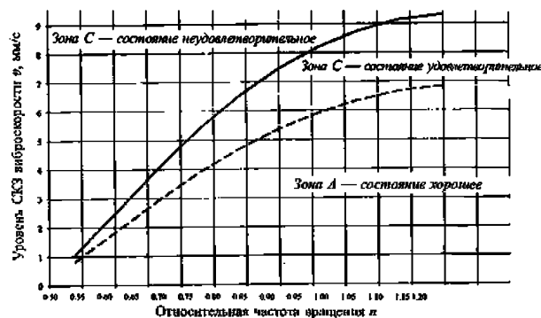
Рис. 9.9.3 Нормы вибрации винторулевых колонок
