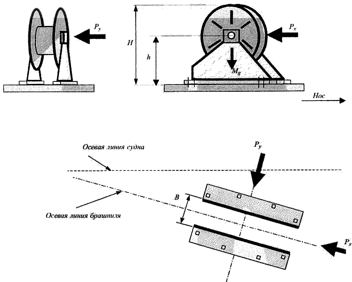
Рис. 6.3.5.3 Направление сил
