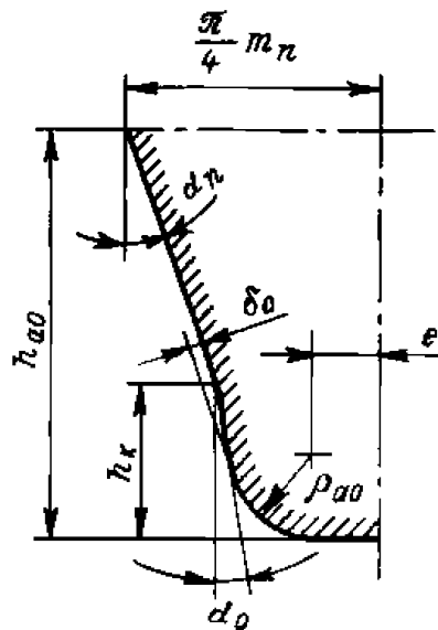
Рис. 4.2.2.7.3.2-3 Исходный производящий контур фрезы с протуберанцем
