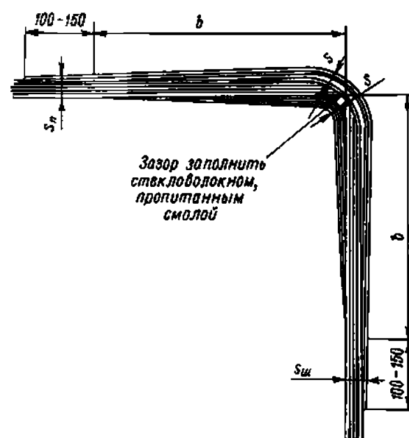
Рис. 1.7.9: s_{нп} — толщина ширстрека; s_n — толщина настила палубы; s — толщина приформовочного угольника; b — 1/2 развернутой ширины угольников
