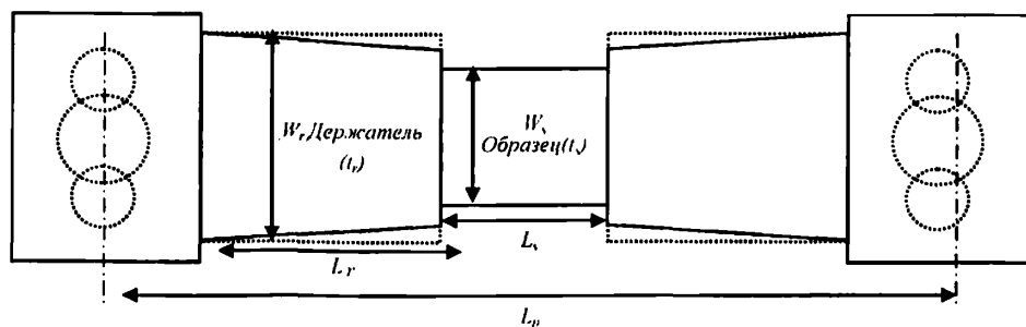
Рис. 3.20.6.2 Схема расположения испытываемого образца, держателя и оснастки
