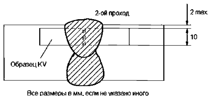
Рис. 4.4.3.2.3 Схема вырезки образцов на ударный изгиб для пробы стыкового соединения, выполненного по двухпроходной технологии сварки
