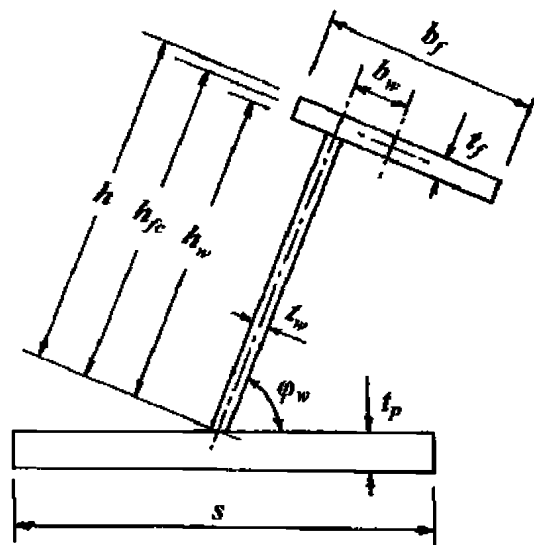
Рис. 1.2.5.7 Геометрия ребра жесткости
