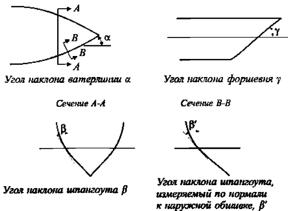
Рис. 1.2.3.2.1.1.1 Определение углов наклона
