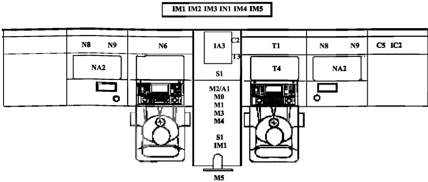
Отдельные рабочие места. Вариант расположения основного оборудования на центральном пульте. Свободный доступ для выполнения функций маневрирования в положении стоя (см. 3.3.3)
