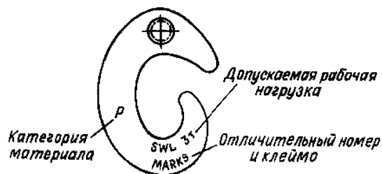
Рис. 11.2.1-1 Маркировка гака
