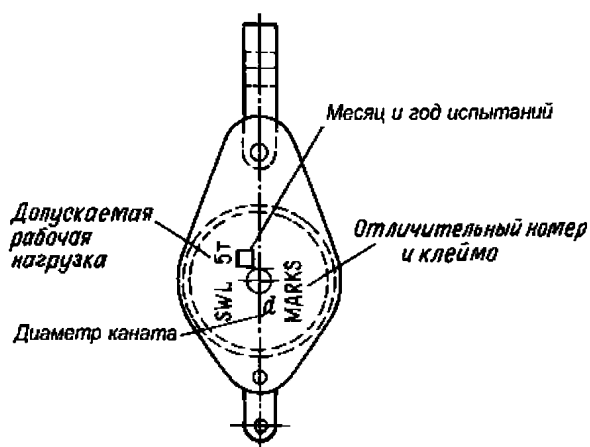
Рис. 11.2.1-5 Маркировка блока
