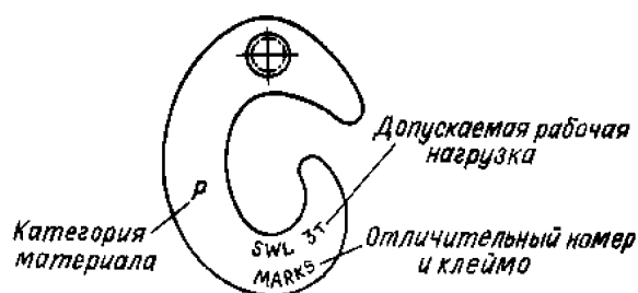
Рис. 11.2.1-1 Маркировка гака
