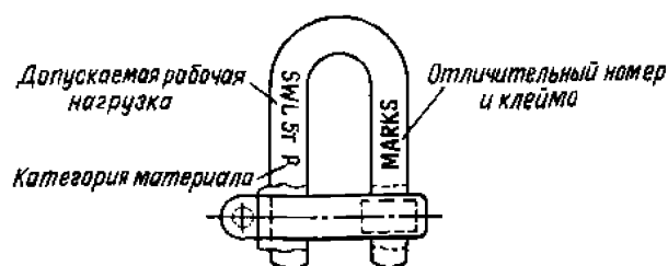
Рис. 11.2.1-3 Маркировка скобы
