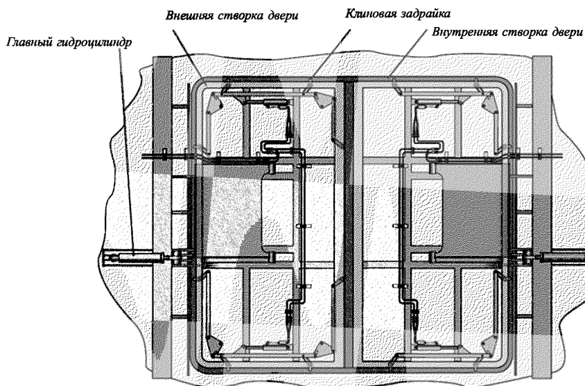
Рис. 32 Бортовaя дверь – двухстворчатая, закрытое положение, вид изнутри
