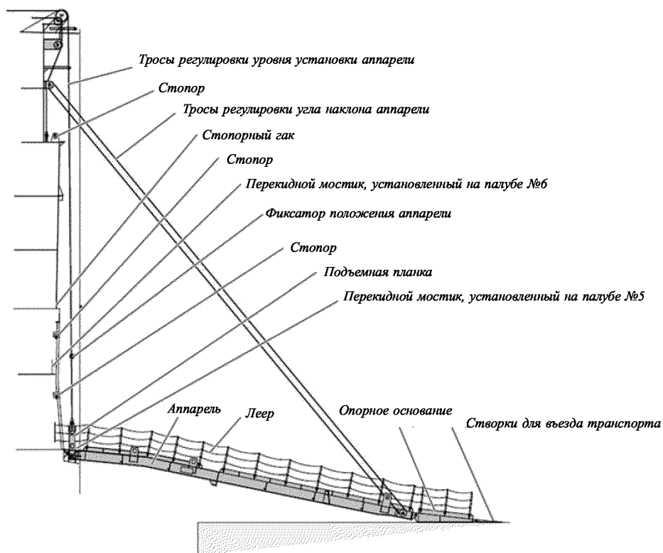
Рис. 38 Бортовая аппарат – вид сбоку
