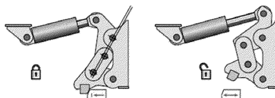
Рис. 17 Клиновая задрайка
