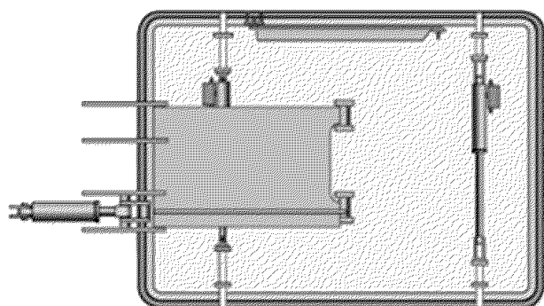
Рис. 25 Бункерный лацпорт – тип 1, в закрытом положении, вид изнутри
