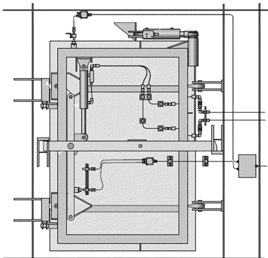
Рис. 36 Лощманская дверь – вид изнутри
