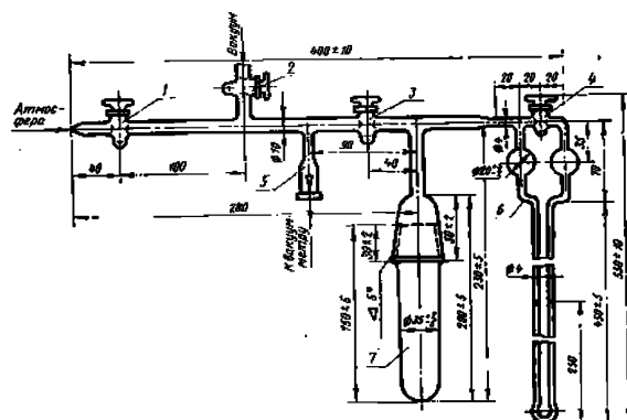
Рис. 5.4.6.5.1 Прибор для определения диффузионного водорода по ГОСТ 23338 метод 2:
