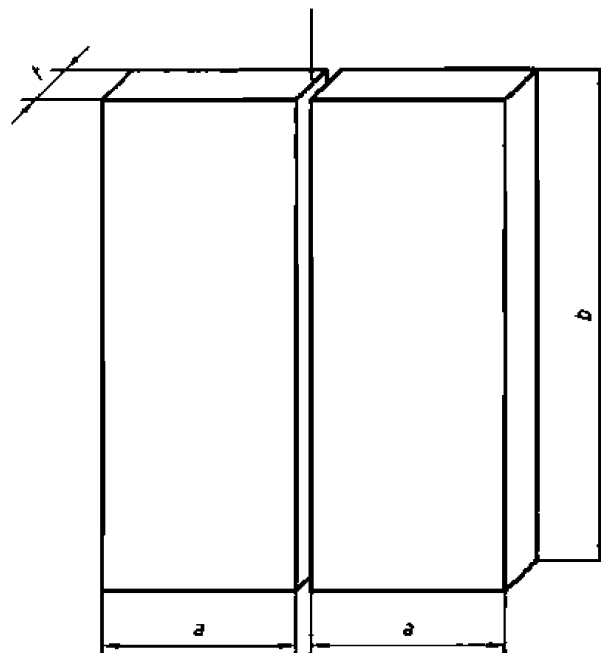
Рис. 8.2.2.4 Проба стыкового соединения листов:
