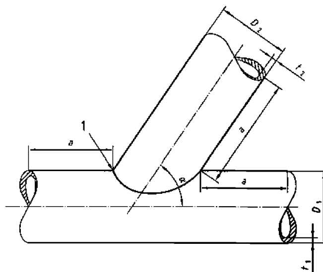
Рис. 8.2.2.7 Проба узла сочленения труб: l – конструктивные элементы подготовки кромок и зазор в соответствии с пСПС; t – толщина основного металла; a \geq 150 мм; D_1 – наружный диаметр основной трубы; D_2 – наружный диаметр присоединяемой трубы; t_1 – толщина металла основной трубы; t_2 – толщина металла присоединяемой трубы; \alpha – угол между осями соединяемых труб
