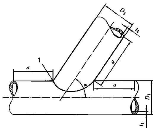
Рис. 6.3.1.6 Проба узла сочленения труб: a \geq 150 мм;
