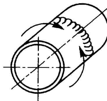
РР: Вертикальное положение (снизу-вверх) труба: неподвижная ось: горизонтальная
