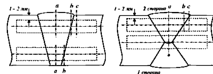
Рис. 6.4.4.4-2 Схема вырезки и расположения надреза на образцах для испытаний на ударный изгиб для технологических процессов сварки с погонной энергией \leq 50 кДж/см: a — надрез по центру шва (WM); b — надрез по линии сплавления (FL); c — надрез по ЗТВ на расстоянии 2 мм от линии сплавления (FL + 2)
