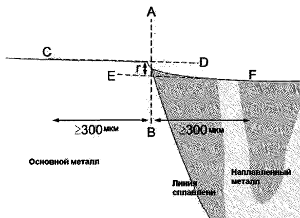
Рис. 2.6.8.3.2.1 Определение глубины коррозии по микрофотоснимку
