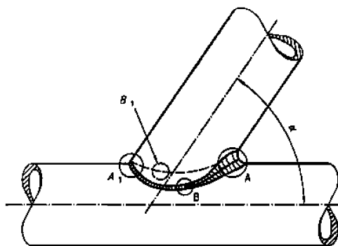
Рис. 8.3.2.1-5 Схема отбора образцов из пробы узла соединения труб:
