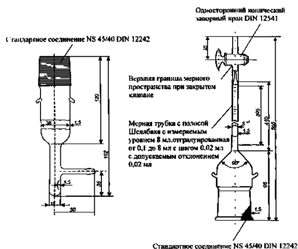
Рис. 5.4.6.6.1-2 Газовая бюретка для определения содержания диффузионного водорода
