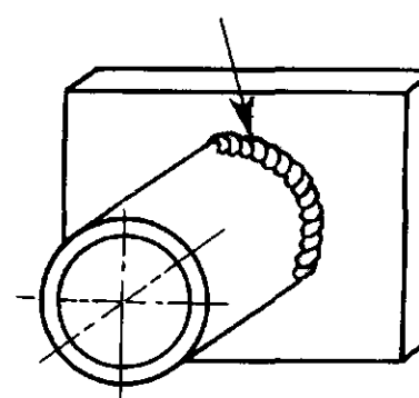
РВ: Горизонтально-вертикальное положение труба: поворачивается ось: горизонтальная
