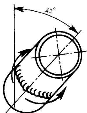
Н-Л045: Наклонное положение (снизу-вверх) труба: неподвижная ось: наклонная
