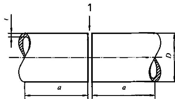
Рис. 6.3.1.3 Проба стыкового сварного соединения труб:
