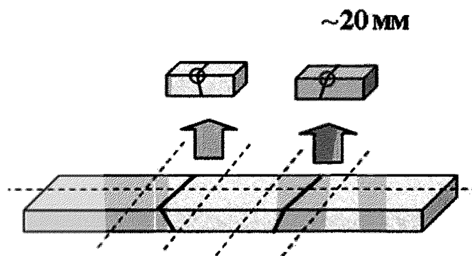
Рис. 2.6.8.3.1.1.1 Схема вырезки образцов
