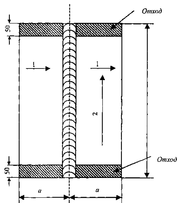
Рис. 6.3.1.2 Проба стыкового сварного соединения листов:
