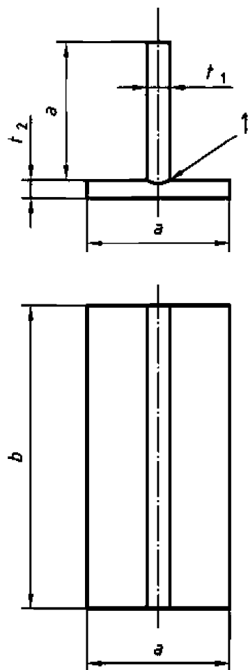
Рис. 8.2.2.6 Проба таврового соединения листов и полуфабрикатов: l – конструктивные элементы подготовки кромок и зазор в соответствии с пСПС; t – толщина основного металла; a \geq 150 мм; b \geq 350 мм
