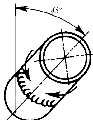
Ж-Л045: Наклонное положение (сверху-вниз) труба: неподвижная ось: наклонная
