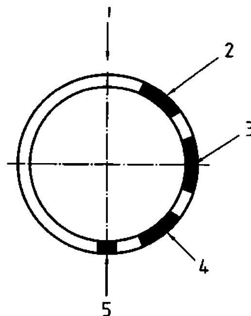
Рис. 8.3.2.1-2 Схема отбора образцов из пробы стыкового соединения труб: 1 – верх (12 часов) неподвижной трубы; 2 – зона для вырезки 1 образца на растяжение и 2 образцов на статический изгиб; 3 – зона для вырезки дополнительных образцов, если требуется; 4 – зона для вырезки 1 образца на растяжение и 2 образцов на статический изгиб; 5 – зона для вырезки 1 макрошлифа и 1 микрошлифа
