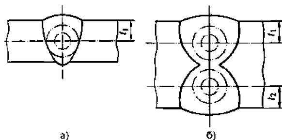
Рис. 6.4.4.1-5 Схема вырезки продольных цилиндрических образцов на растяжение:
