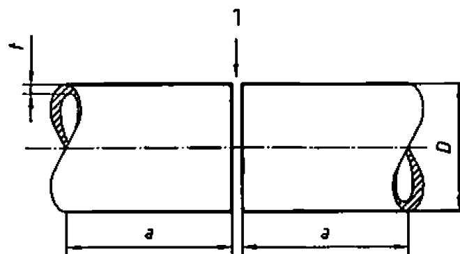
Рис. 8.2.2.5 Проба стыкового соединения труб:
