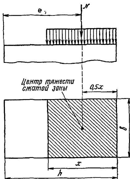
Рис. 4. Расчетная схема для бетонного элемента прямоугольного сечения
