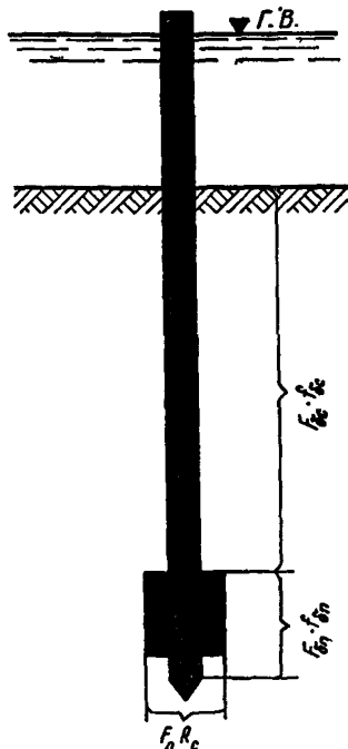
Расчетная схема определения несущей способности забивной сваи с уширенной пяткой
