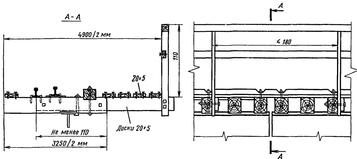
Рис. 2. Тротуары и перила на пролетных строениях с деревянными поперечинами (вариант с удлинением поперечин досками; размеры даны в сантиметрах)
