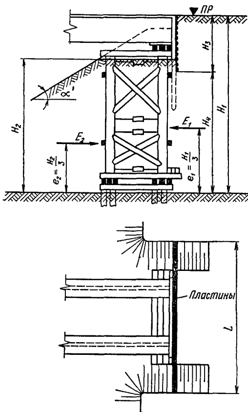
Рис. 1. К определению горизонтального давления на устои собственного веса грунта подходной насыпи
