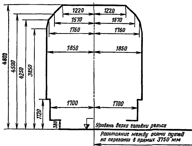
Рис. 2. Условный габарит приближения строений 1-СМ-О
