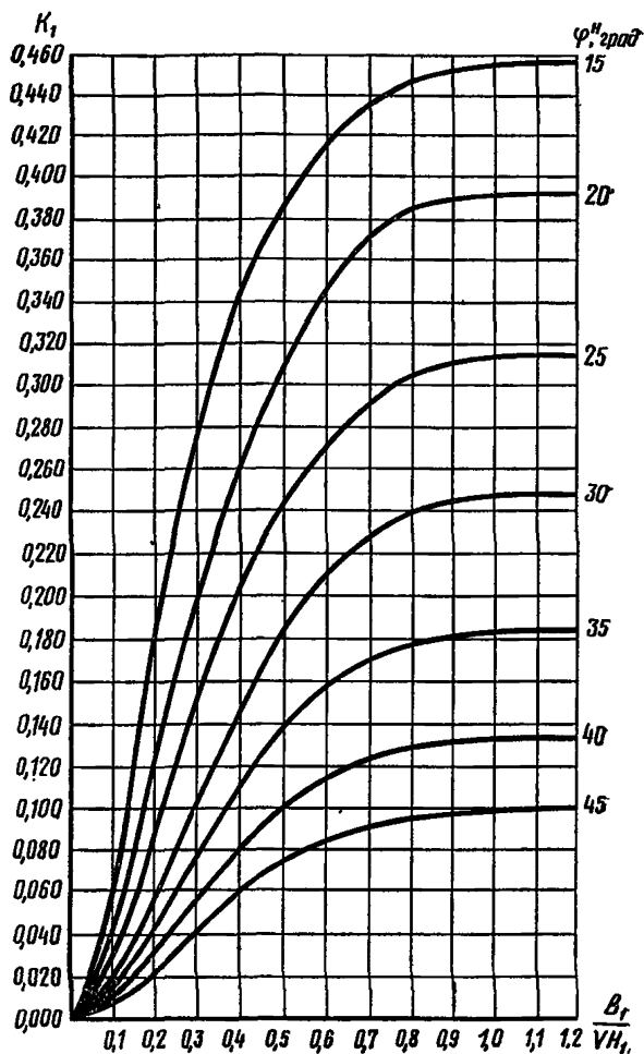
Рис. 2. График зависимости коэффициента K_1 от угла внутреннего трения \varphi^n и отношения \frac{B_1}{VH_1}
