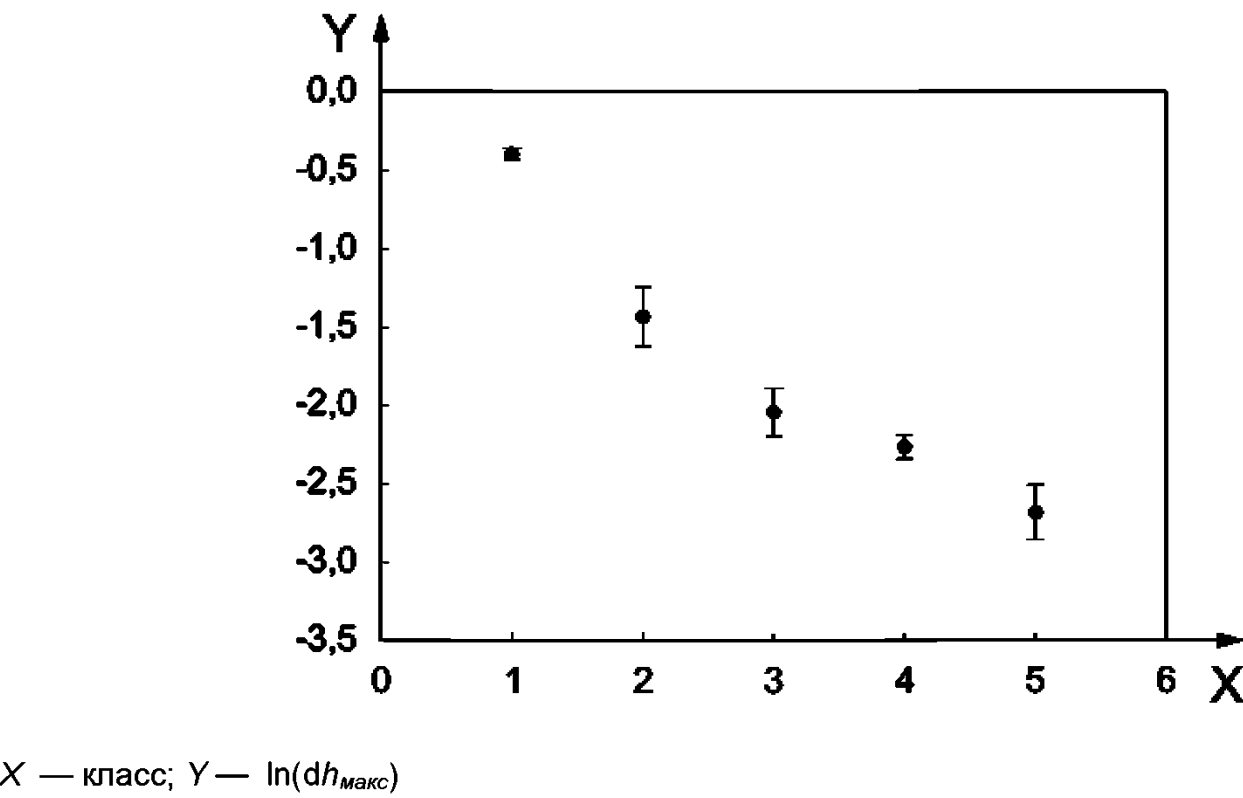
Рисунок В.14 — Соотношение между классом и преобразованным dh_{\text{макс}}
