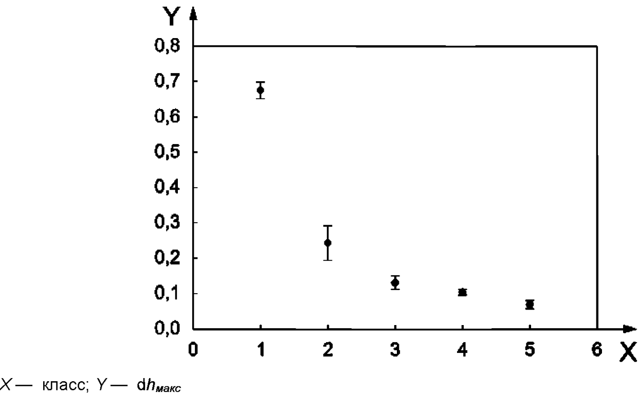
Рисунок В.13 — Соотношение между классом и исходным dh_{\text{макс}}
