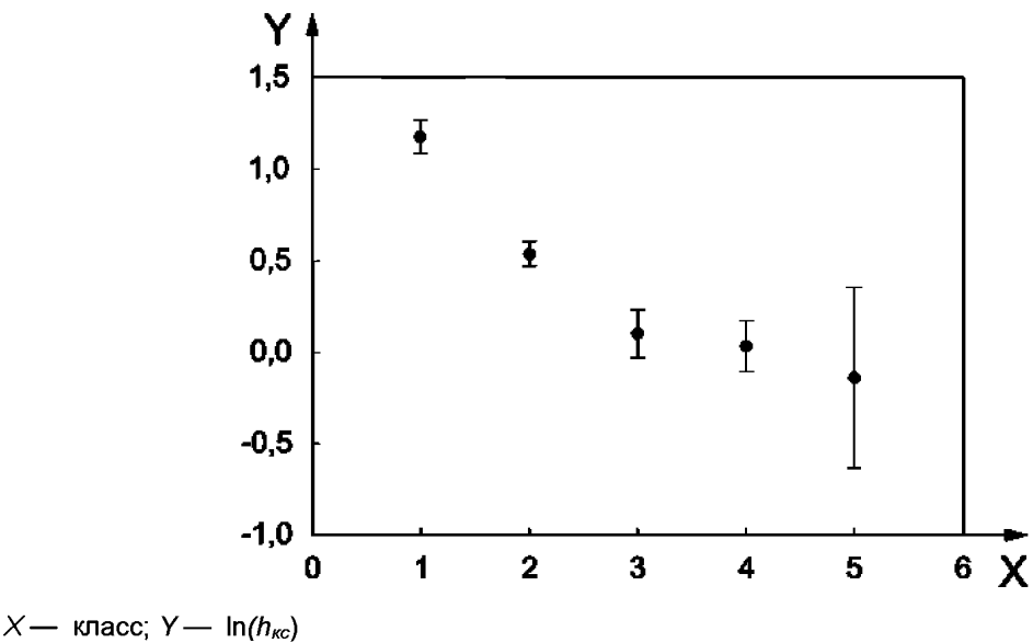
Рисунок В.8 — Соотношение между классом и преобразованным h_{\text{макс}}
