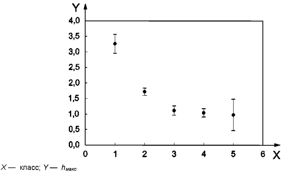
Рисунок В.7 — Соотношение между классом и исходным h_{\text{макс}}
