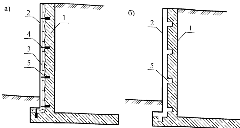
Рисунок 7.1 – Нарращивание обоймы с внешней грани подпорных стен:
