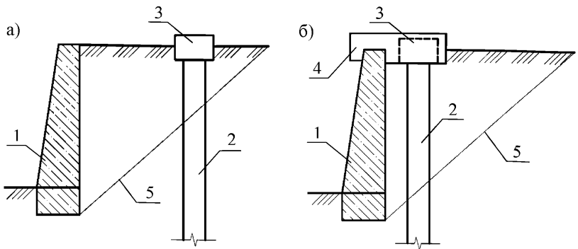
Рисунок 7.11 – Устройство свайного поля с верховой стороны существующего сооружения: а) отсечение части призмы обрушения;
