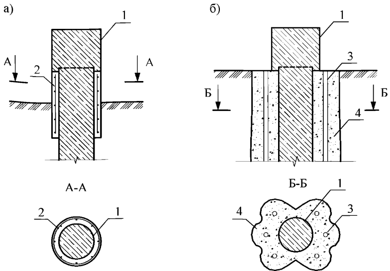
Рисунок 7.3 – Усиление стволов свай удерживающих сооружений:
