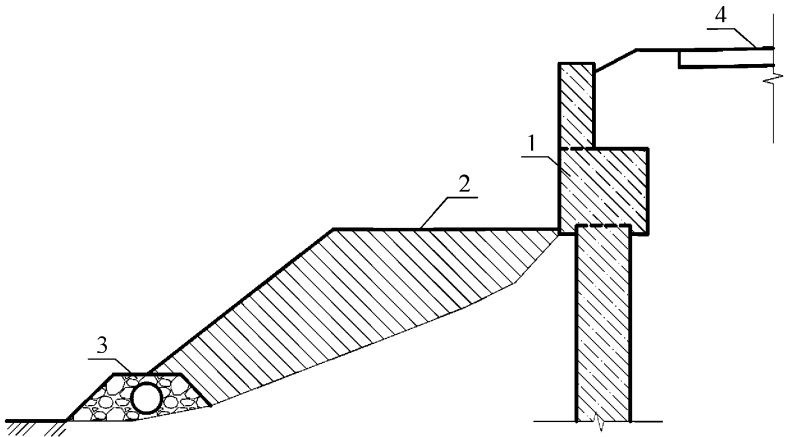
Рисунок 7.5 – Усиление низового сооружения контрбанкетом
