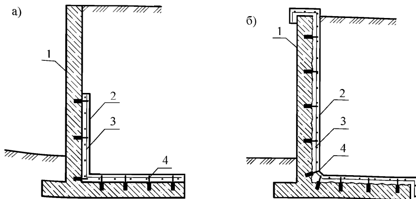
Рисунок 7.2 – Нарращивание железобетонной обоймы в растянутой зоне:
