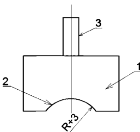
Рисунок 4.6 – Гладилка для обработки поверхности продольной подливки:
