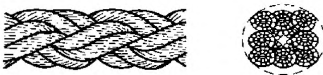
Рисунок 3 — Конфигурация 8-рядного плетеного каната (тип L)
