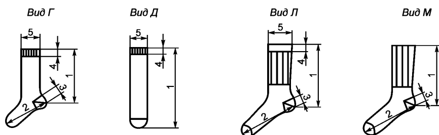
Рисунок 2 — Полу чулки (гольфы)
