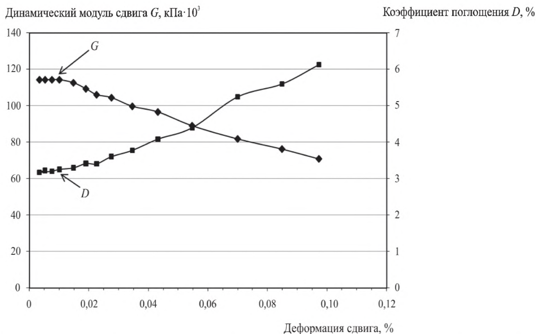
Рисунок Л.3 – Пример зависимости упругих и диссипативных характеристик глинистого грунта от уровня сдвиговых деформаций по результатам одного испытания на резонансной колонке
