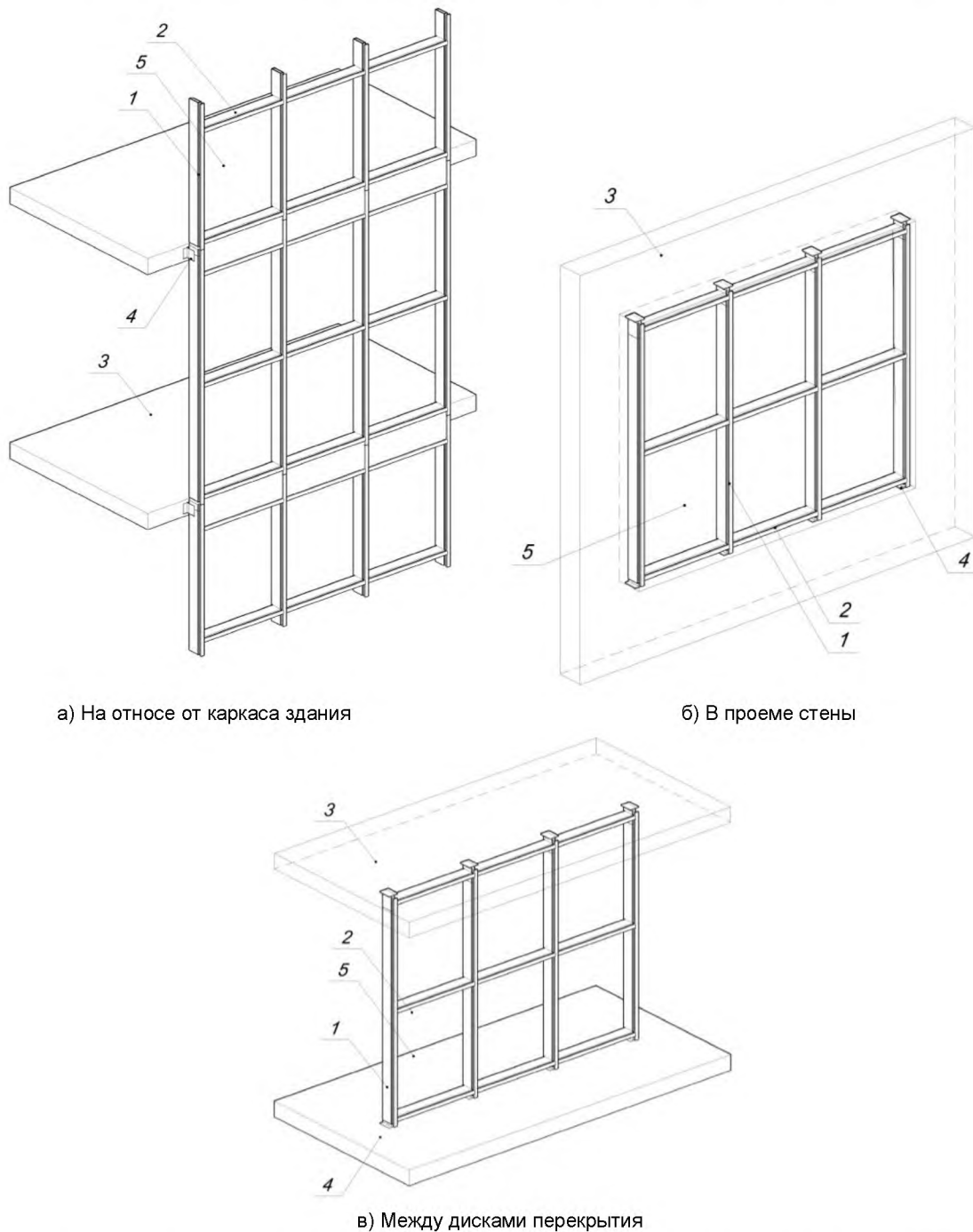
Рисунок А.1 – Стоечно-ригельная конструкция
