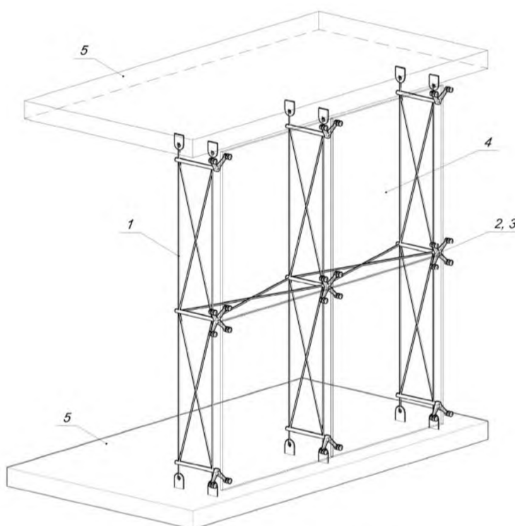
б) Вантовая конструкция из стержней
