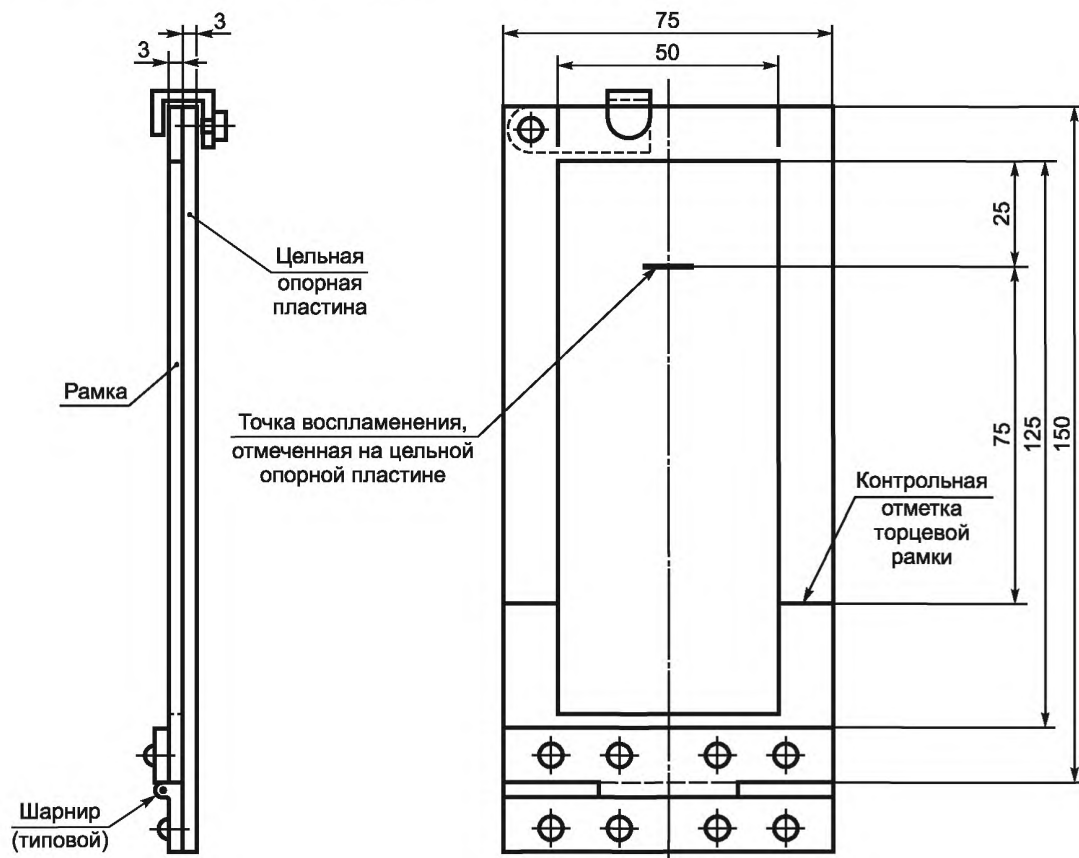
Рисунок 1 — Держатель образца
