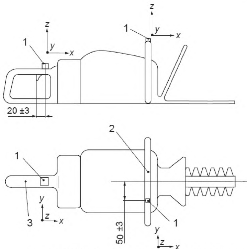
1 – акселерометр; 2 – передняя рукоятка; 3 – задняя рукоятка
