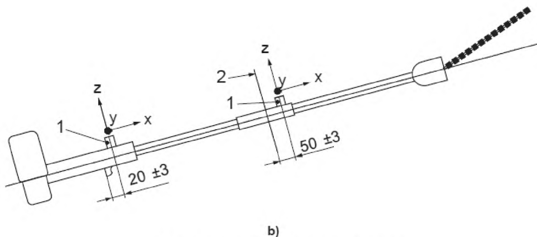
Рисунок D.3 – Направления измерений и точки крепления акселерометров на машинах дальней досягаемости
