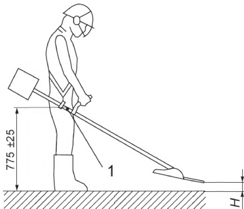
1 – точка подвеса
