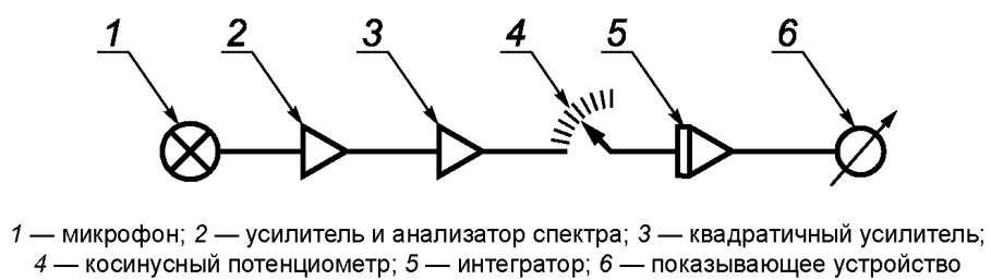
Рисунок G.3 — Пример цепи преобразования сигнала микрофона
