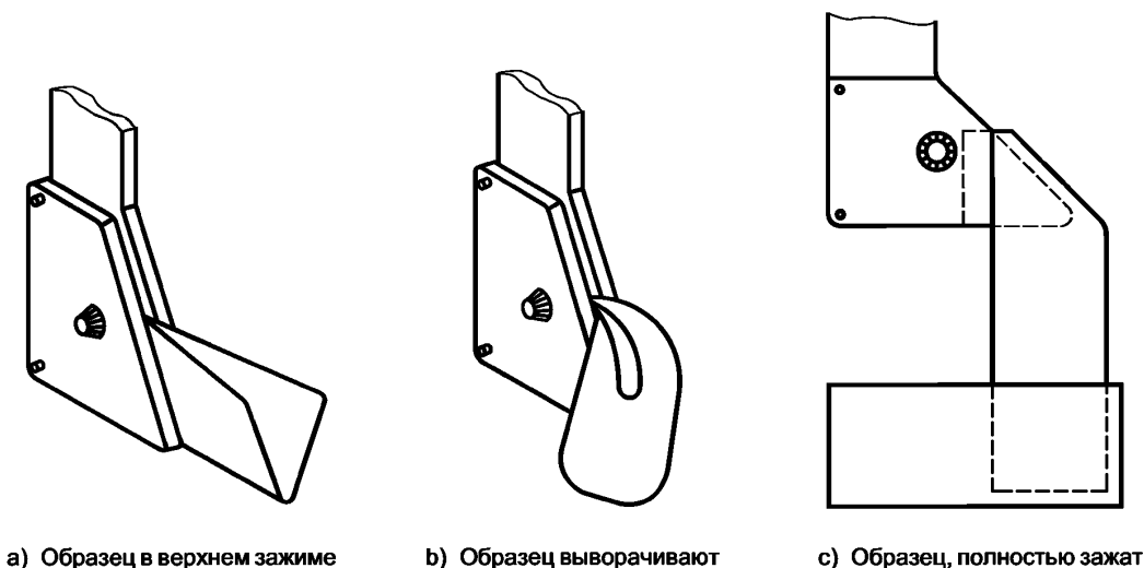
Рисунок 2 — Загрузка образца
