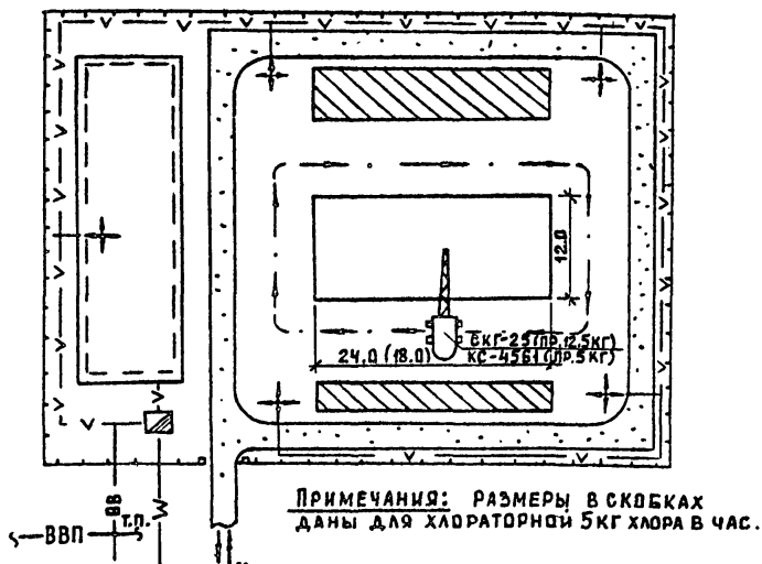
РИС.1 СХЕМА СТРОЙГЕНПЛАНА
