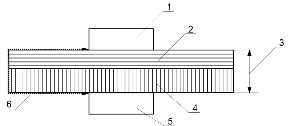
1 — проводящая часть 1; 2 — слой изоляции 1; 3 — требований к минимальному расстоянию через изоляцию нет; 4 — слой изоляции 2; 5 — проводящая часть 2; 6 — зазор и путь утечки (равны)
