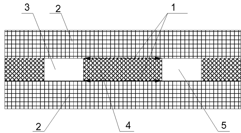
1 — потенциальный зазор и путь утечки вдоль скрепленного стыка; 2 — изоляционный слой; 3 — проводящая часть 1; 4 — изоляционный компаунд; 5 — проводящая часть 2
