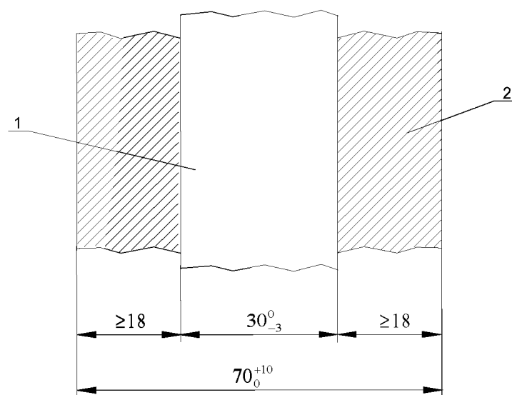
1 — металлическая фольга; 2 — изоляционный материал
