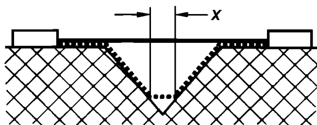
Рисунок F.3 — V-образная канавка
