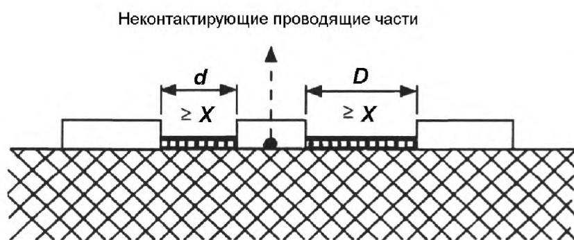
Рисунок F.13 — Интервал, несоединенная проводящая часть
