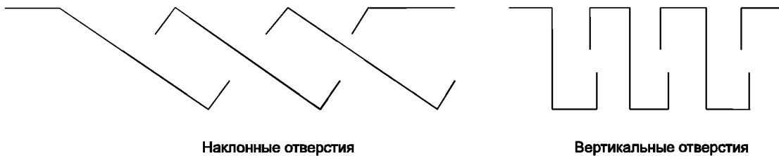
Рисунок 4В — Примеры поперечного сечения конструкции отверстий
