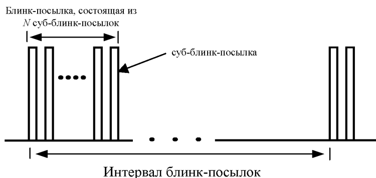
Рисунок 5 — Радиоинтерфейс DSSS
