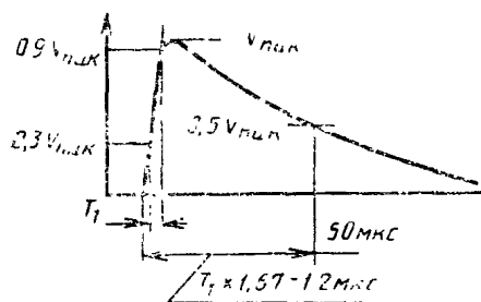
Рисунок Н26.8.1 — Форма волны при разомкнутой цепи
