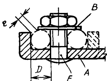
Болтовые зажимы
