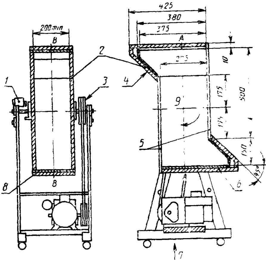
1—автоматический счетчик падений, останавливающий вращение после определенного числа оборотов; 2—стенка толщиной 19 мм или другой подходящий вариант; 3—приводной клиновидный ремень или другой подходящий вариант; 4—облицовка из материала с низким коэффициентом трения; 5—окна для наблюдения (могут быть съемными); 6—стенка толщиной 19 мм или другой подходящий вариант; может быть съемной; 7—барабан, вращающийся по часовой стрелке; 8—поверхность падения из стали толщиной 3 мм; 9—центральная точка пересечения осей
