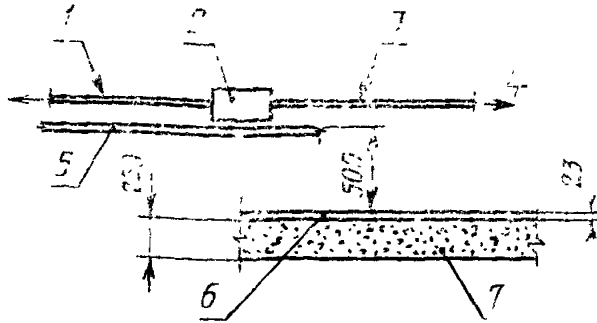
1—выходной гибкий кабель; 2—образец; 3—входной гибкий кабель; 4—напряжение (по таблице пункта 12.7.2); 5—стеклянная поверхность; 6—твердая древесина (толщина 23 мм); 7—бетон (толщина 250 мм)
