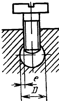
Зажим без прижимной пластины
