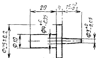
Рисунок 1 — Испытательный стержень
