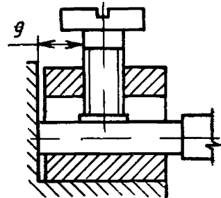
Зажим с прижимной пластиной
