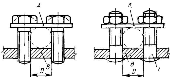
А—прокладка; В—закрепленная часть; С—штифт; D—пространство для провода
