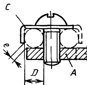
Винтовые зажимы
