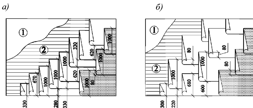
Рисунок 5.4 – Раскладка рулонных материалов:
