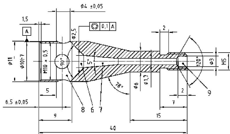
d) Трубка горелки
