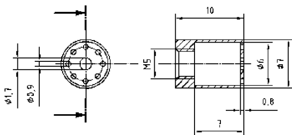
c) Стабилизатор пламени
