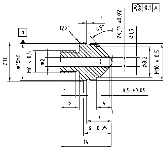
b) Газовый жиклер
