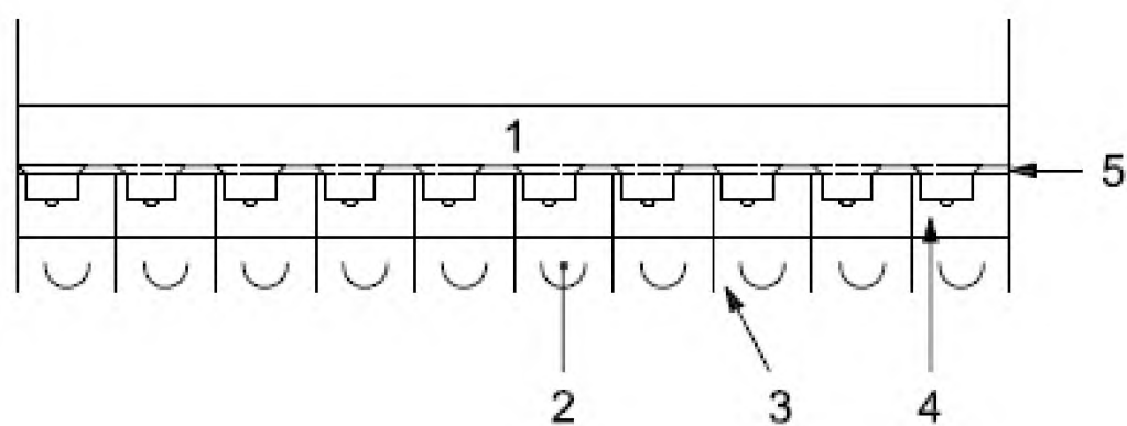
1 — вспомогательный лоток; 2 — индивидуальные испытательные кабины; 3 — разделительная перегородка между испытательными кабинами; 4 — люк; 5 — стена с окошками для передачи проб
