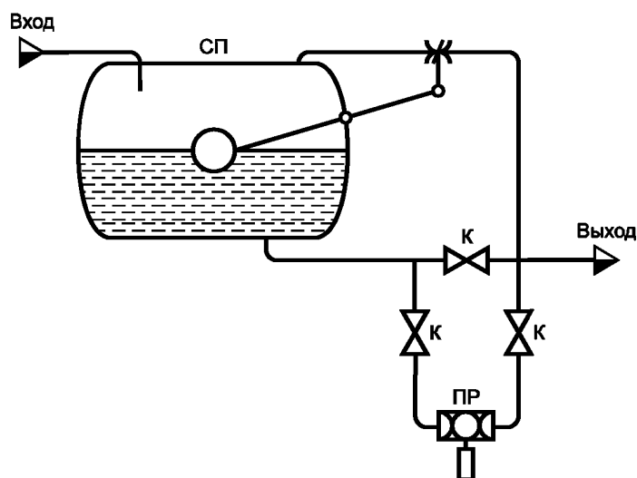
Рисунок А.7 — Средства отбора проб сырой нефти из потока нефтегазовой смеси с контуром отбора проб и депульсатором на входе
