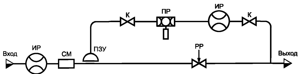
Рисунок А.4 — Средства отбора проб сырой нефти из потока нефтеводогазовой смеси, расположенные в трубопроводе
