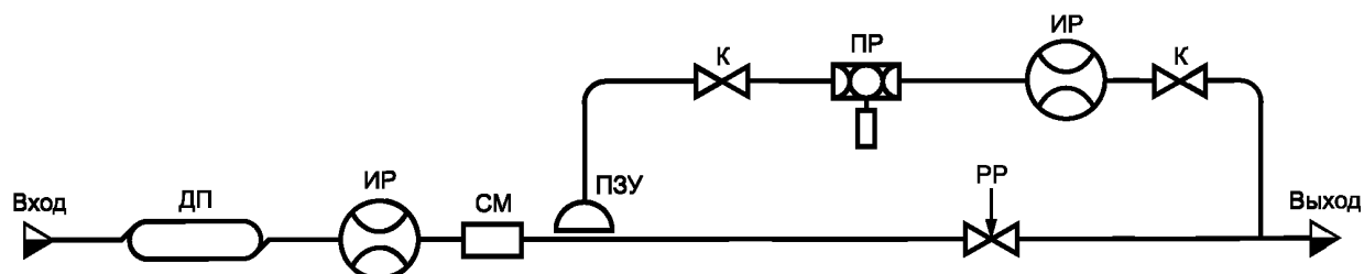
Рисунок А.6 — Средства отбора проб сырой нефти из потока нефтегазовой смеси, расположенные в трубопроводе с депульсатором на входе
