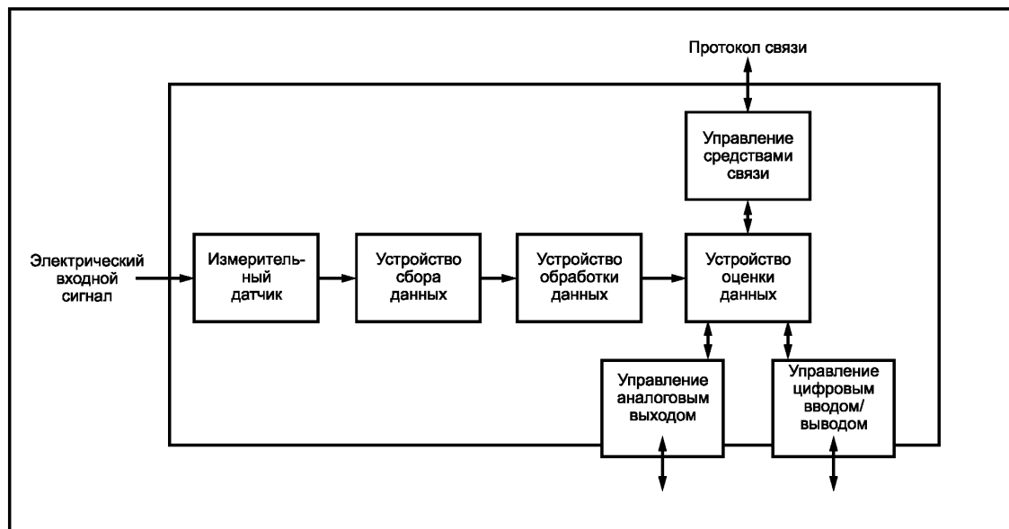
Рисунок 1 — Структура преобразователя
