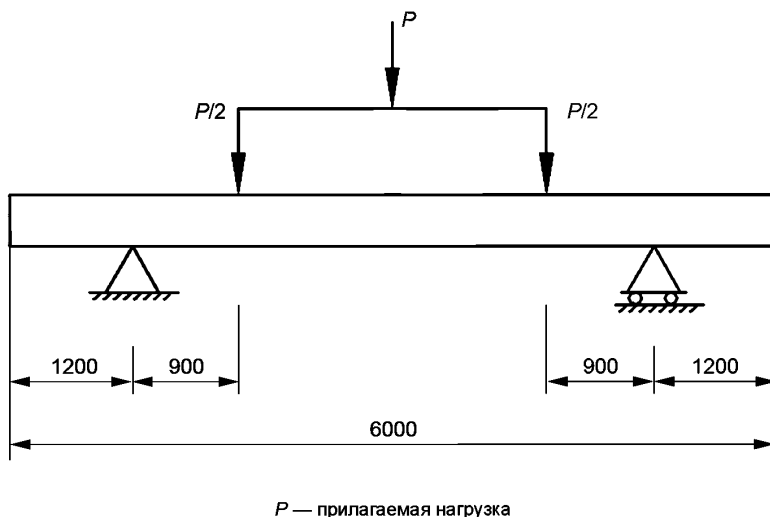
Рисунок 3 — Схема нагружения плиты длиной 6 м
