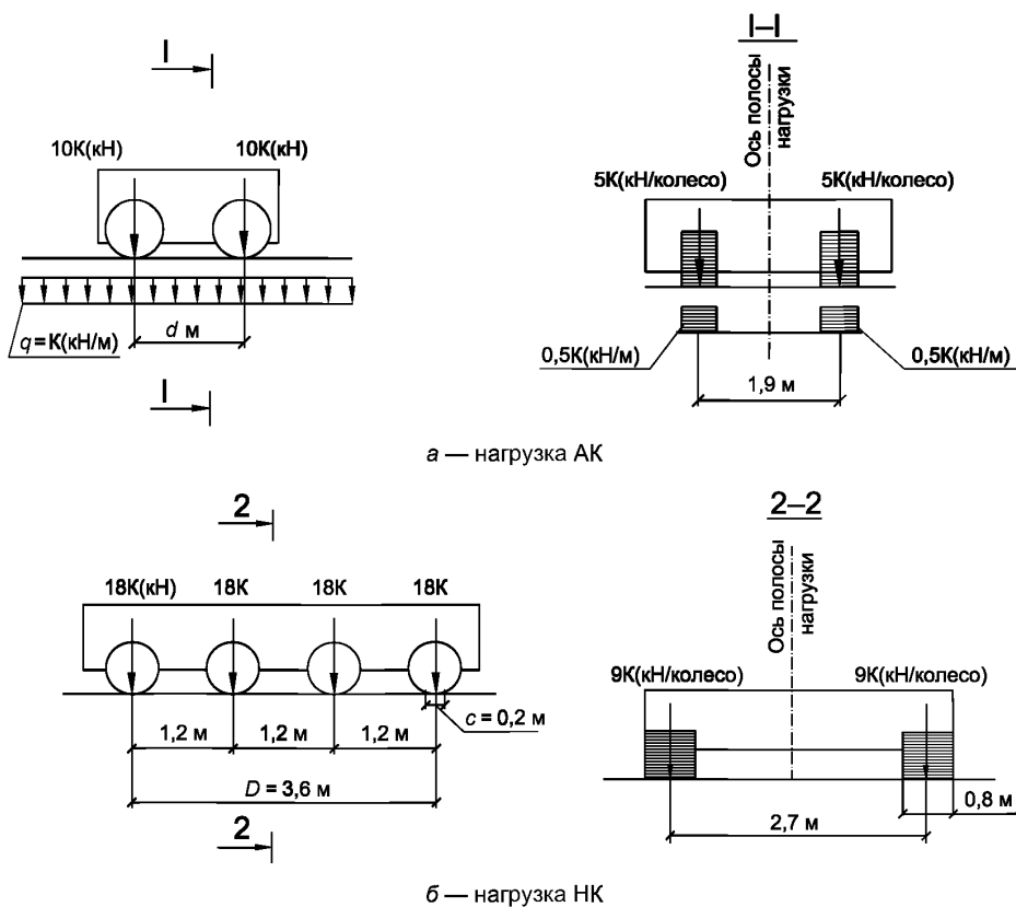
Рисунок 1 — Схемы нормативных нагрузок для расчета дорожной одежды, земляного полотна, подпорных стен и мостовых сооружений
