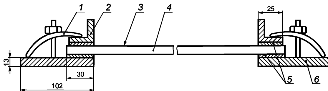
1 — зажим; 2 — внутренняя рама; 3 — поверхность остекления 900 \times 1100 мм; 4 — образец; 5 — резина; 6 — наружная рама
