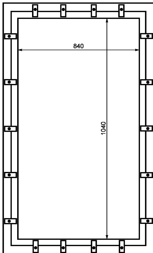
Рисунок В.2 — Наружная рама
