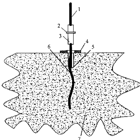
1 – направляющий стержень; 2 – ограничитель; 3 – штуцер; 4 – фанерное основание; 5 – шпур; 6 – трещина; 7 – тело бетона
