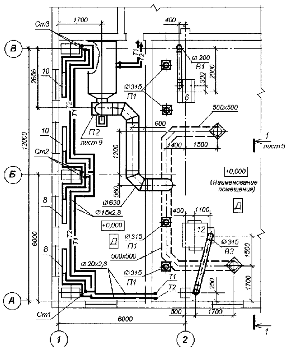
План 2-2
