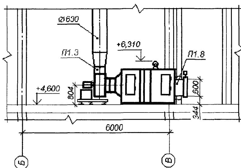
Разрез 1-1
