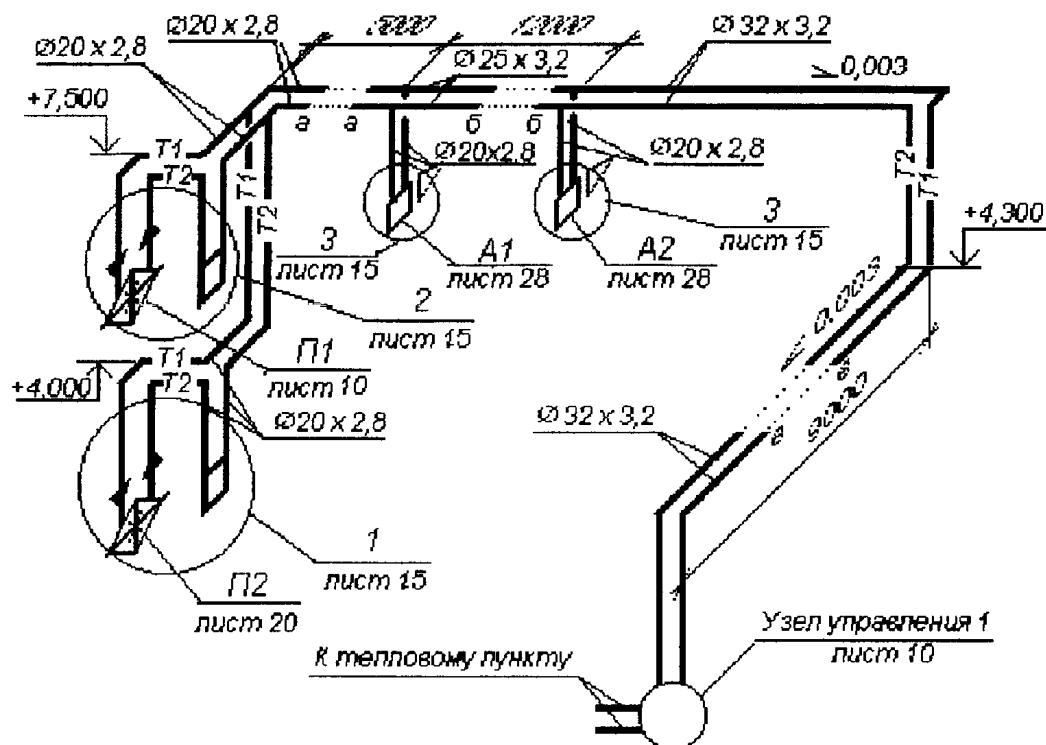
Система теплоснабжения установок П1, П2, А1, А2
