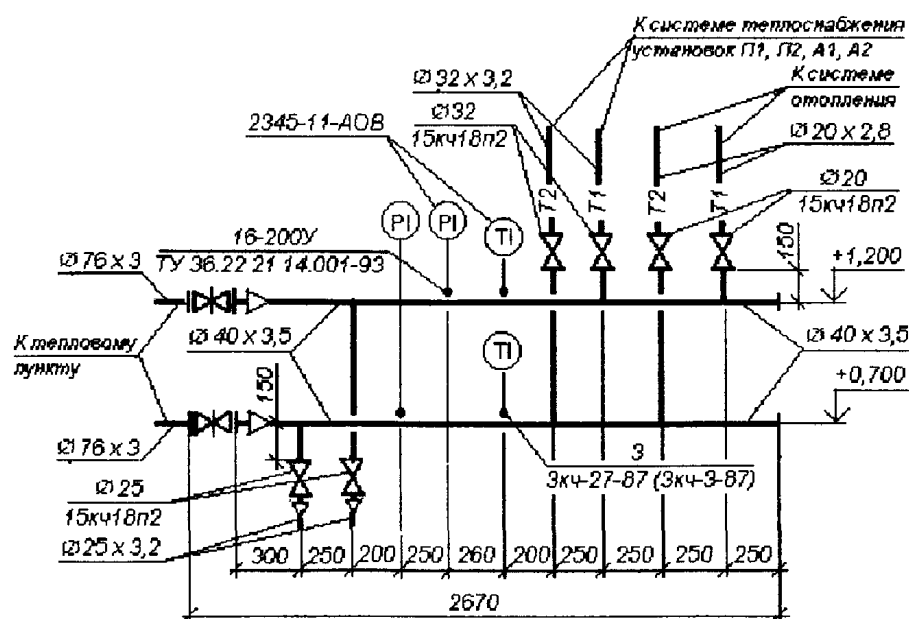
Узел управления 1
