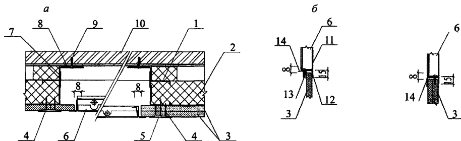
a – горизонтальный разрез; б – вертикальный разрез
