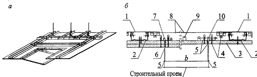
а – общий вид подвесного потолка со смотровым ревизионным люком; б – разрез подвесного потолка со смотровым ревизионным люком (на примере подвесного потолка, конструкция 4 таблица 13)
