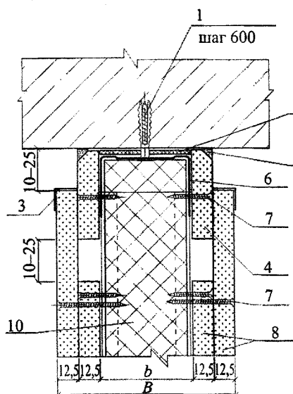
Рисунок 3 – Присоединение перегородки с обшивками из гипсокартонных или гипсоволокнистых листов к потолку
