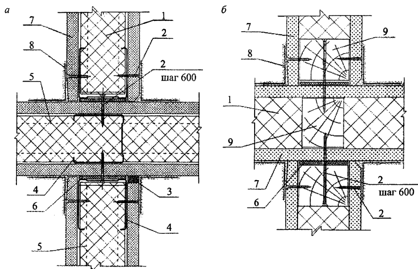
а – перегородки с металлическим каркасом и вставкой из металлического профиля; б – перегородки с деревянным каркасом и вставкой из деревянного профиля
