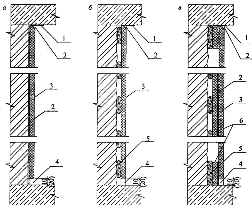
а – крепление гипсокартонных листов на ровное основание; б – крепление гипсокартонных листов на основание с неровностью до 20 мм; в – крепление гипсокартонных листов на основание с неровностью свыше 20 мм
