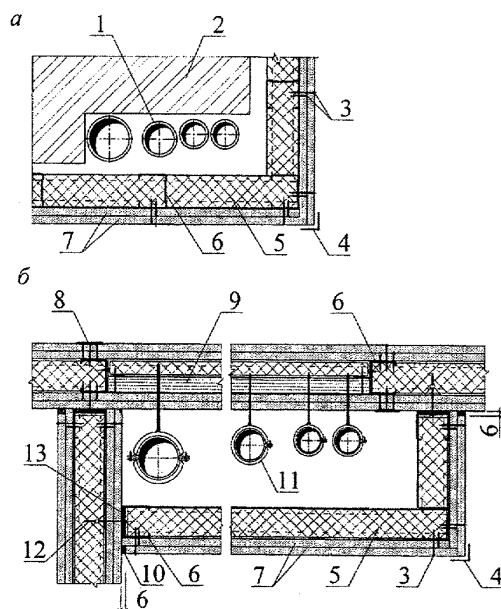
а – у несущей стены; б – у перегородки
