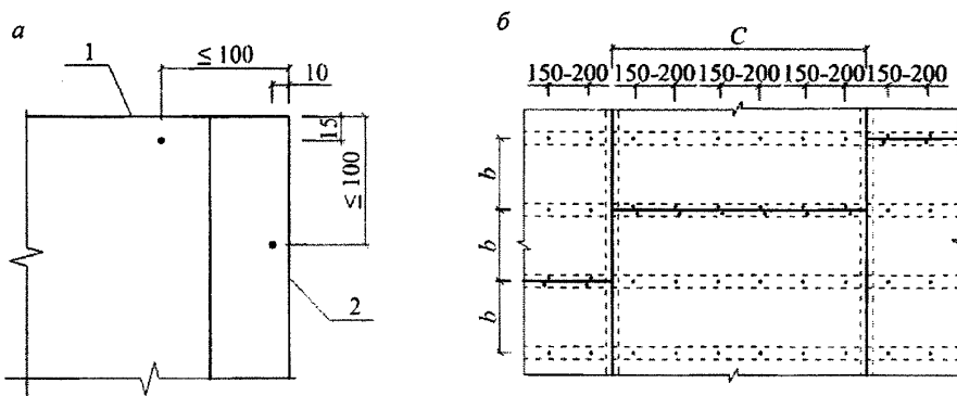
а – схема расположения самонарезающих винтов на краях гипсокартонных листов; б – схема закрепления гипсокартонных или гипсоволокнистых листов к каркасу с помощью самонарезающих винтов
