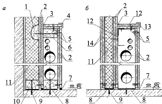
а – размещенных вдоль капитальной стены; б – вдоль перегородки
