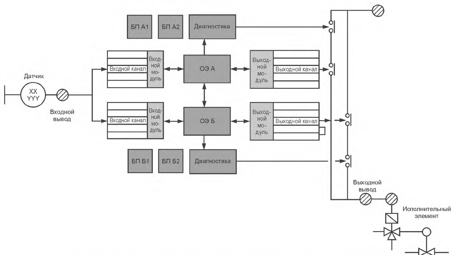
Рисунок В.6 — Два обрабатывающих элемента (ОЭ) с двумя входами/выходами, с межпроцессорной связью, с внешними сторожевыми таймерами и логикой срабатывания 2oo2D
