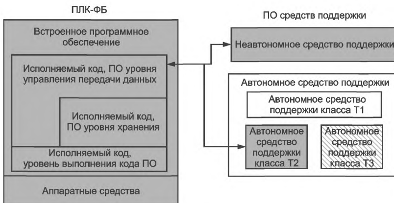
Рисунок 5 — Связь ПЛК-ФБ с инструментальными средствами
