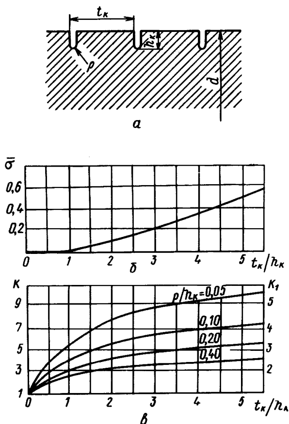
а — схематическое изображение вала с канавками; б — зависимость относительных напряжений \bar{\sigma} на поверхности вала от размеров термокомпенсационных канавок; в — концентрация напряжений на изгиб K , на кручение и сдвиг K_1
