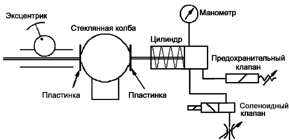
Рисунок С. 1 — Схематическое изображение испытательной установки
