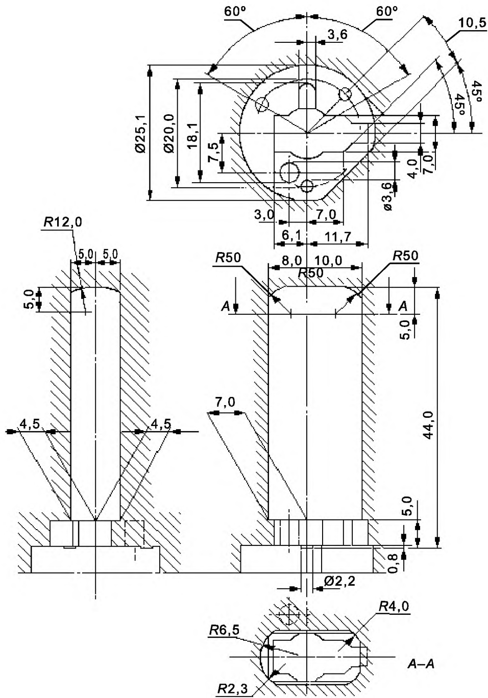
Рисунок F.2 — Наибольшие контуры ламп накаливания категории Н1
