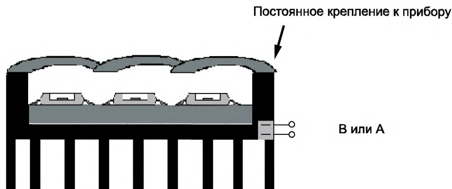
Рисунок 5 — Пример незаменяемого светодиодного источника света
