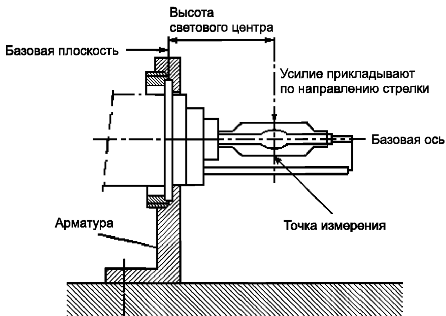
Рисунок Е.1 — Схема испытательной установки
