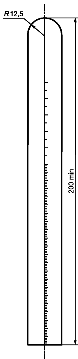
Рисунок D.1 — Градуированный стержень для определения длины презерватива
