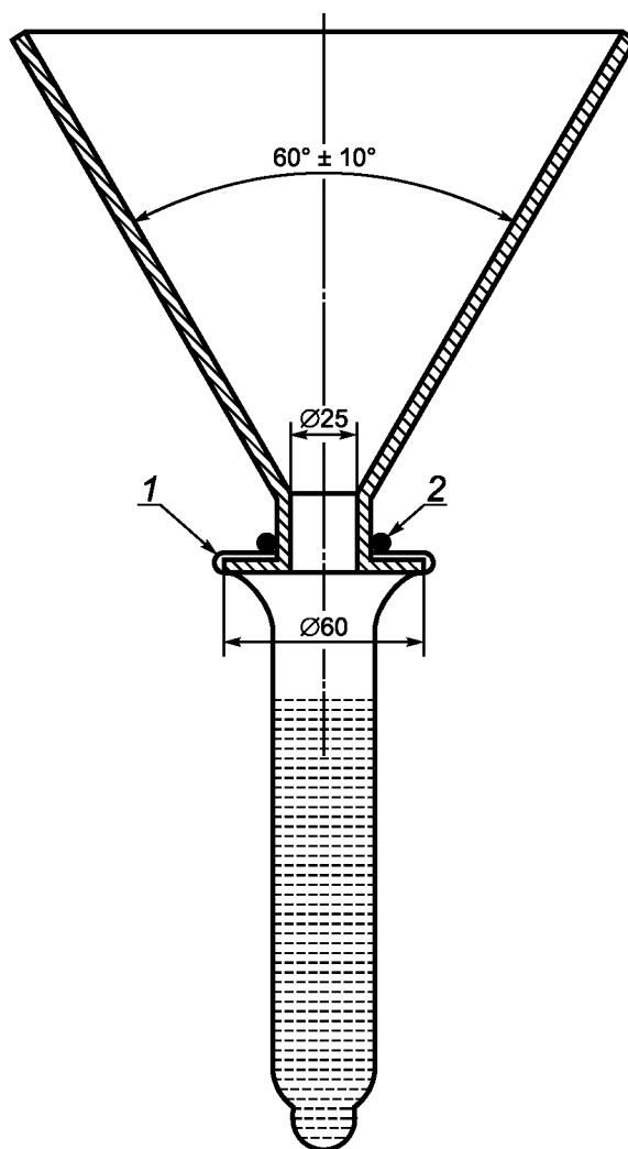
1 — закругленная кромка; 2 — резиновое кольцо
