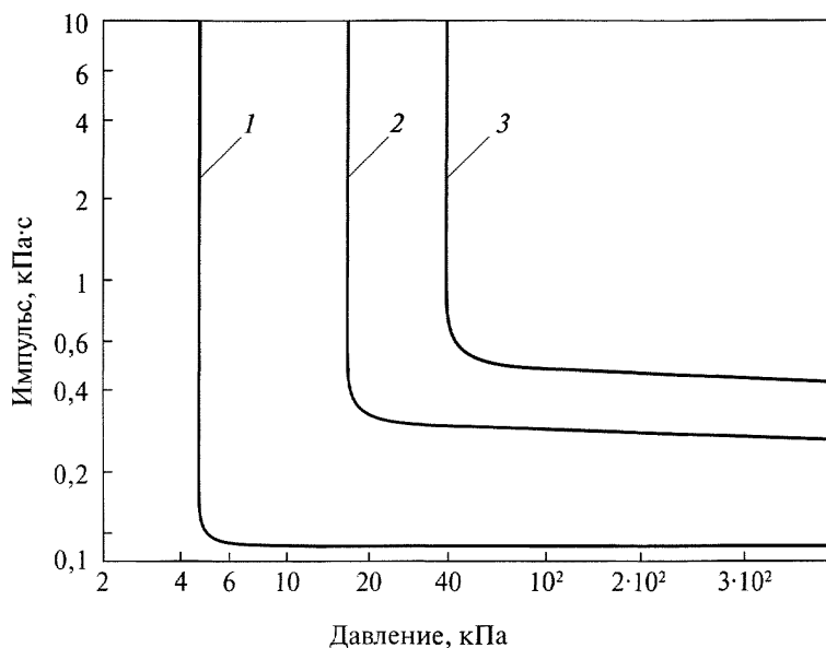
Рис. 2. P-I диаграмма для оценки уровня разрушения промышленных зданий:
