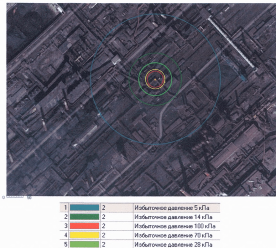
Рис. 5-2. Зоны распространения ударной волны при взрыве ТВС
