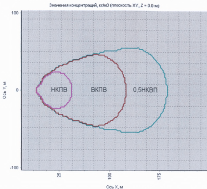
Рис. 5-3. Сечение зоны, ограниченной НКПВ, 0,5НКПВ и ВКПВ плоскостью z = 0 (в направлении по ветру) при выбросе пропана
