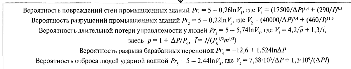
Рис. 3-1. Алгоритм расчета последствий аварийных взрывов топливно-воздушных смесей
