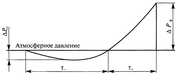
Рис.1. Характерный профиль ударной волны
