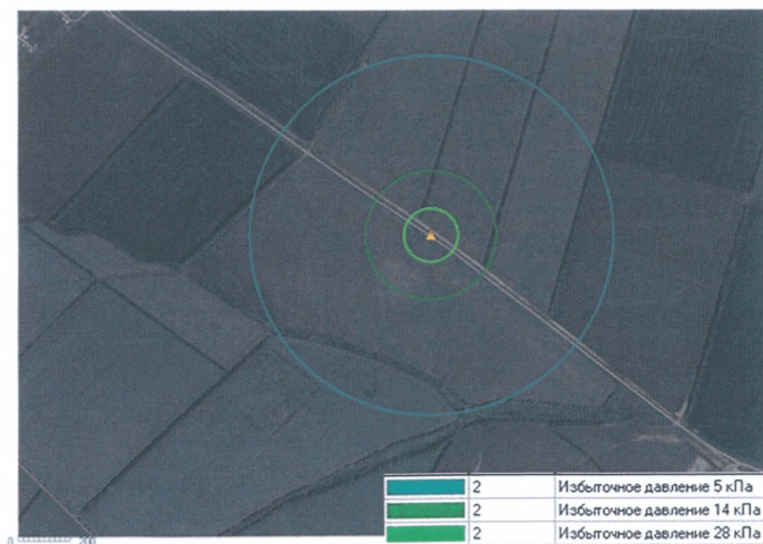
Рис. 5-1. Зоны распространения ударной волны при взрыве ТВС
