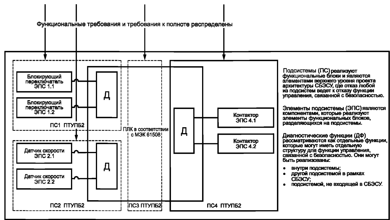
Рисунок В.7 — Архитектура СБЭСУ с диагностическими функциями, встроенными в подсистему 3
