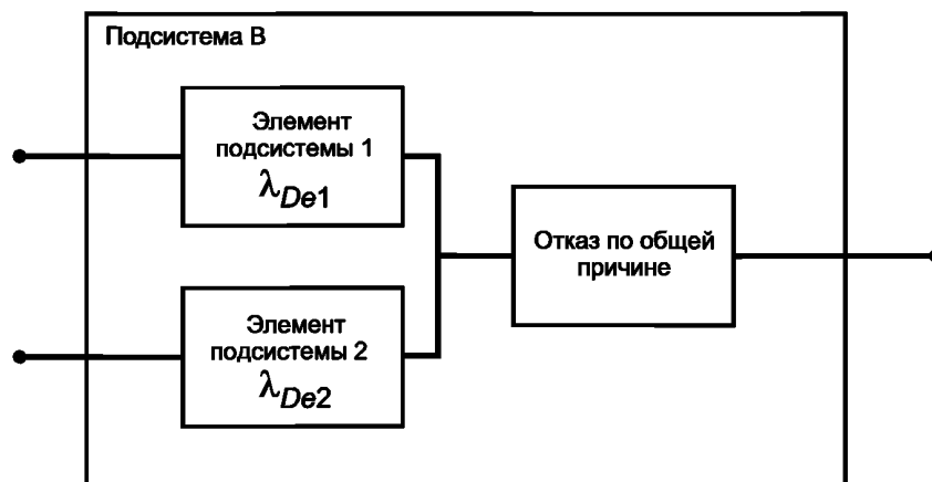
Рисунок 7 — Логическое представление подсистемы типа В
