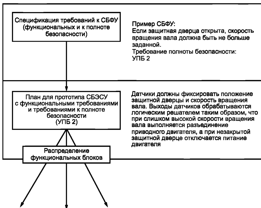
Рисунок В.4 — Декомпозиция в структуру функциональных блоков
