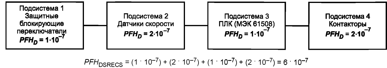
Рисунок В.8 — Оценка PFH_D для СБЭСУ
