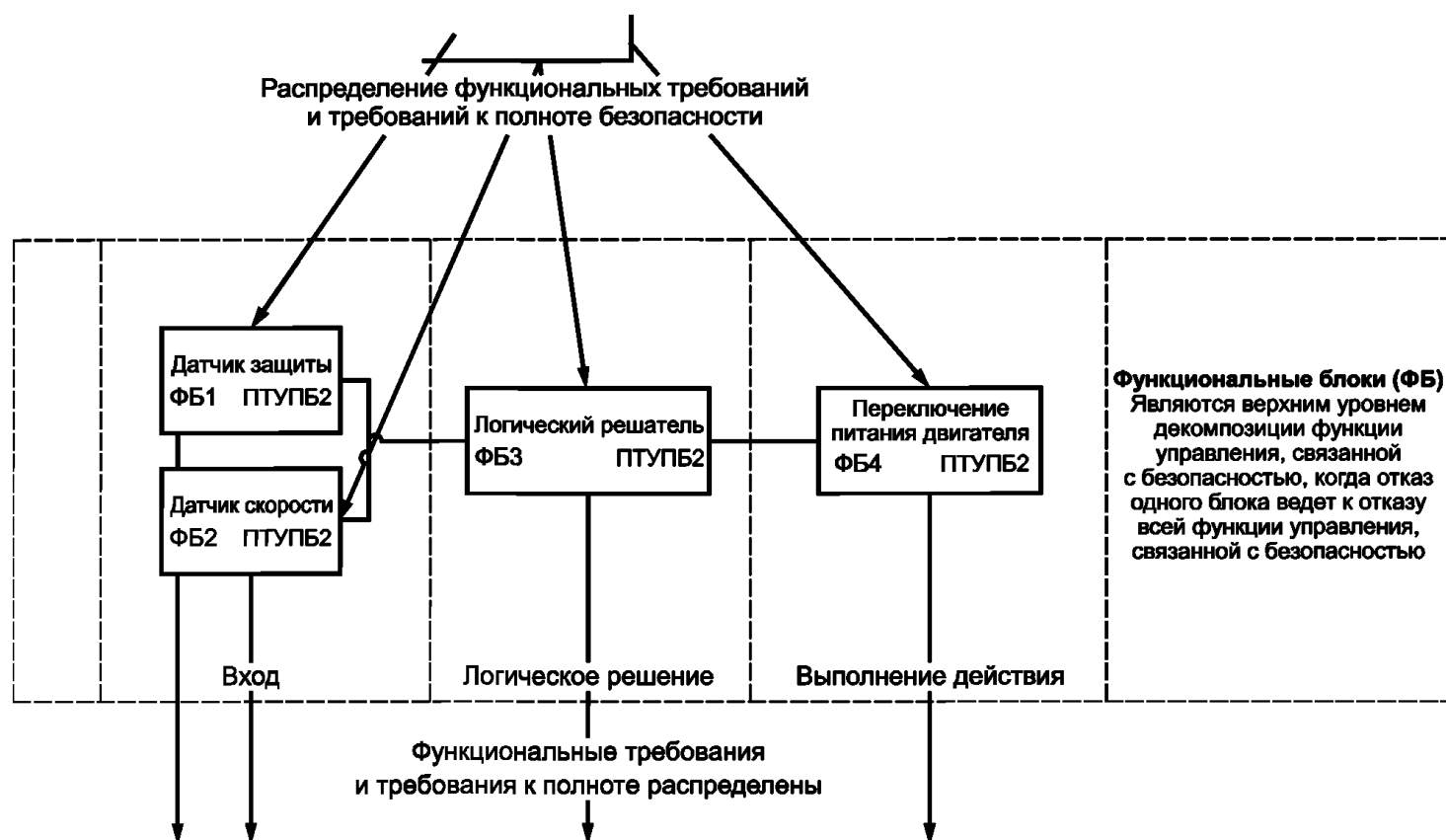
Рисунок В.5 — Начальная концепция архитектуры СБЭСУ
