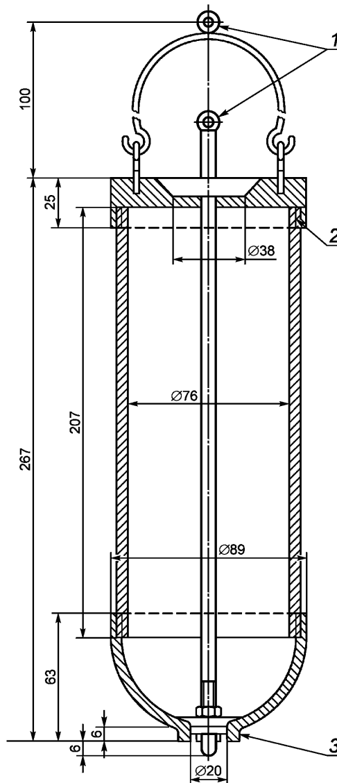
Рисунок 1 — Глубинный пробоотборник
