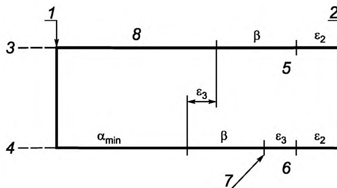
1 — сигнал останова; 2 — контроль торможения; 3 — рабочее давление; 4 — минимальное давление; 5 — ОУ; 6 — УУ; 7 — точка останова при минимальном давлении; 8 — \alpha (угол срабатывания)
