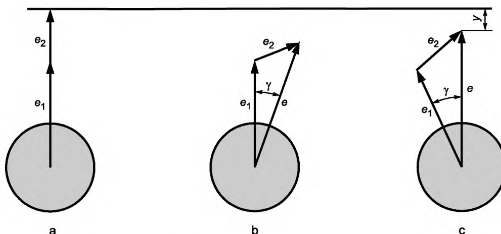
Рисунок Е.2 — Положение эксцентриковой втулки относительно вала
