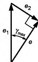
Рисунок Е.3 — Максимальный угол поворота узла поворотных кулачков \gamma_{\max}
