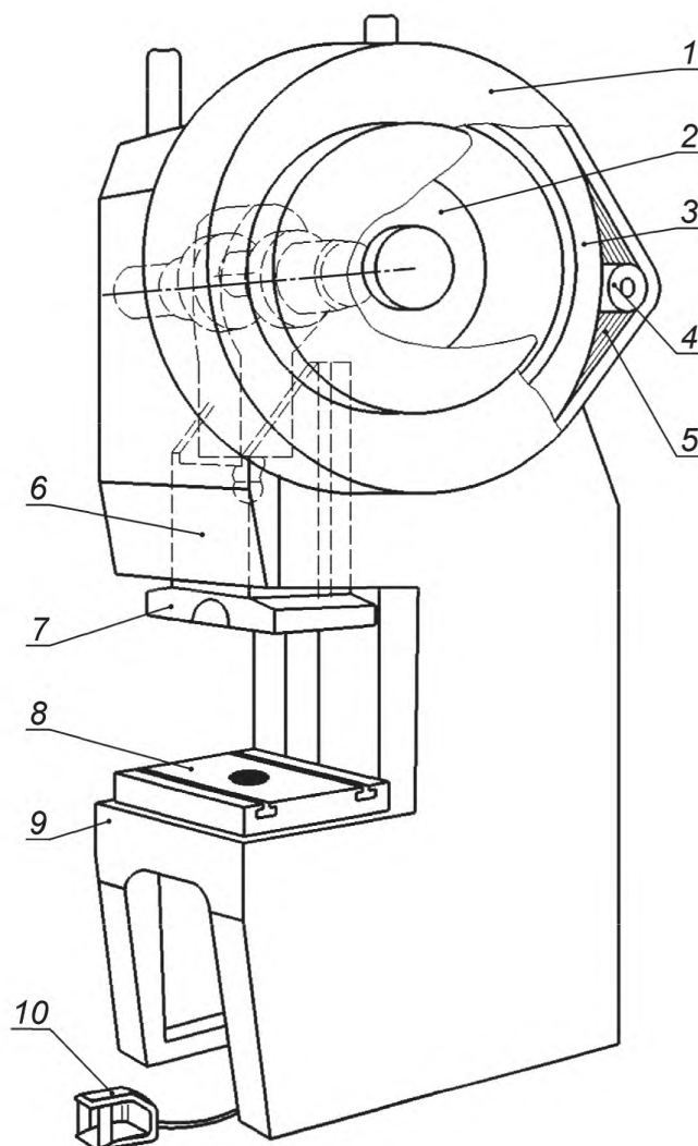
1 — ограждение маховика; 2 — муфта-тормоз; 3 — маховик; 4 — шкив мотора; 5 — ремень; 6 — ползун; 7 — фланец ползуна, держатель штампа; 8 — подштамповая плита; 9 — стол; 10 — педаль
