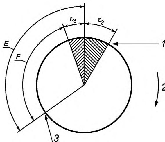
1 — контроль торможения; 2 — направление вращения; 3 — сигнал останова; E — угол при рабочем давлении; F — угол при минимальном давлении; \varepsilon_2 — безопасный интервал контроля торможения (интервал контролируемого перебега), в градусах; \varepsilon_3 — разница между углом при рабочем давлении и углом при минимальном давлении, в градусах
