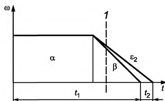
Рисунок F.1 — Отношение между временем срабатывания t_1 , углами срабатывания \alpha и торможения \beta
