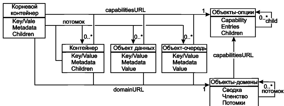
Рисунок 4 – Модель объекта CDMI
