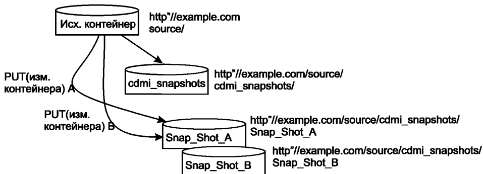
Рисунок 9 – Структура снимка состояния контейнера
