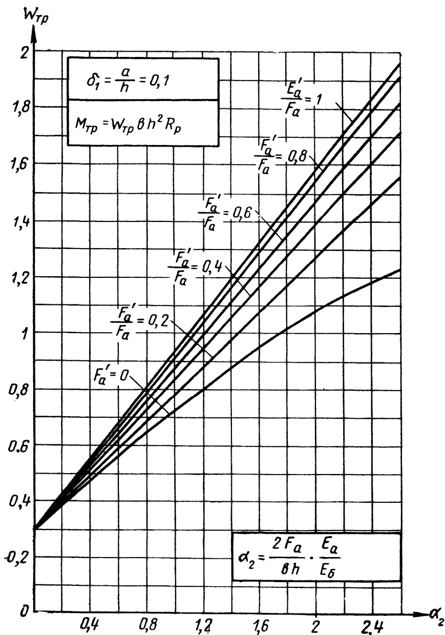
График 2. Значения коэффициента W_{тр} для определения момента появления трещин в изгибаемых элементах прямоугольного сечения при \delta_1 = 0,1
