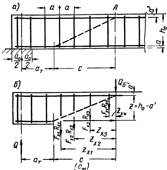
Рис. 3. К расчету изгибаемых элементов по косым сечениям
