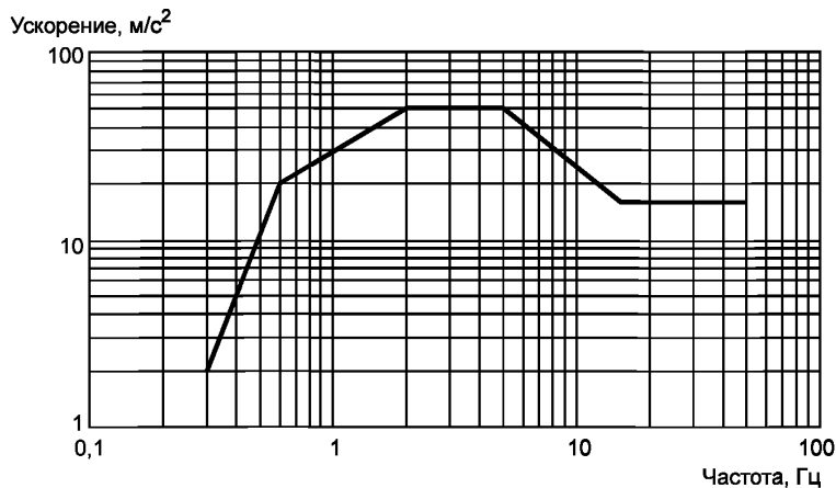
Рисунок 3 — ТСО для тестового сигнала (коэффициент демпфирования 2 %)
