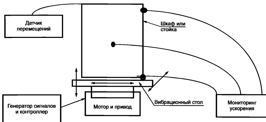
Рисунок 2 — Структурная схема испытания
