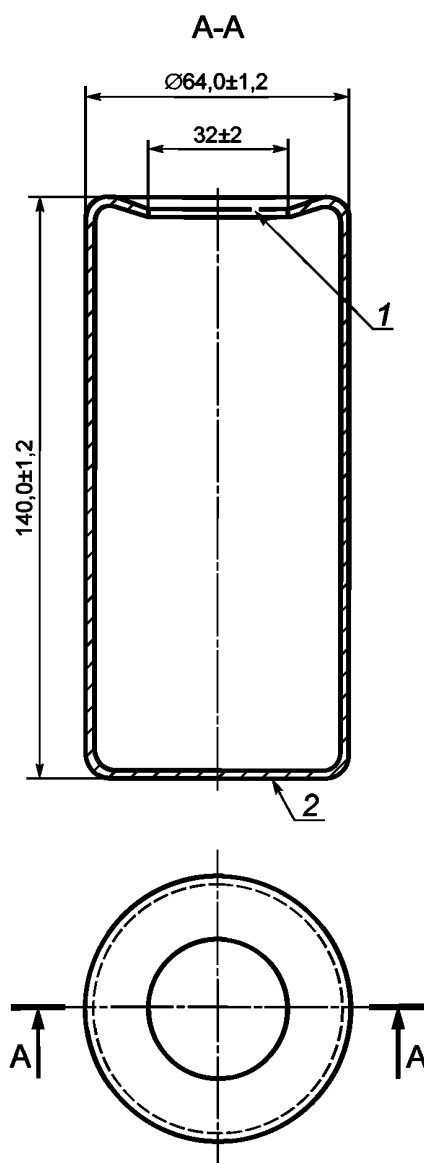
Рисунок 4 — Стекланный контейнер с горловиной, направленной внутрь
