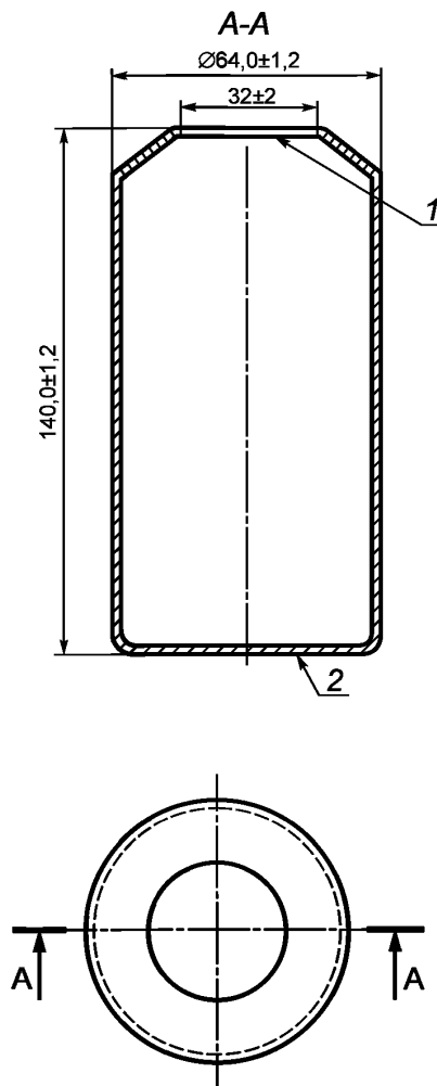
Рисунок 5 — Стекланный контейнер с горловиной, направленной наружу
