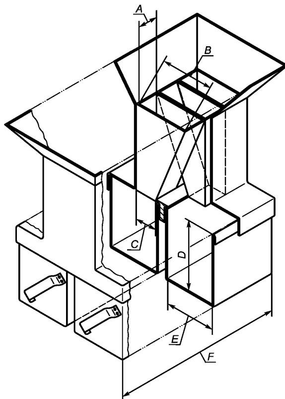
Рисунок А.2 — Пример механического делителя пробы
