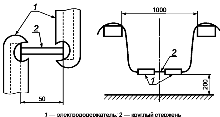
Рисунок 1 — Компоновка испытания на повышение температуры
