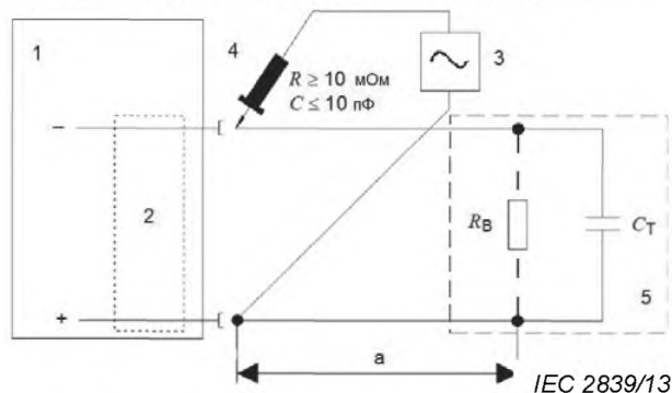
1 — источник тока для сварки или резки; 2 — устройство для зажигания и стабилизации дуги; 3 — осциллограф; 4 — высоковольтный щуп; 5 — нагрузка в максимально компактном исполнении; а — максимально короткий соединительный провод
