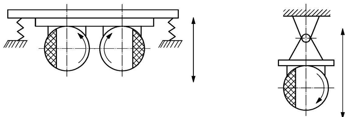
а) Два внешних вибратора во вращающихся противоположных направлениях
