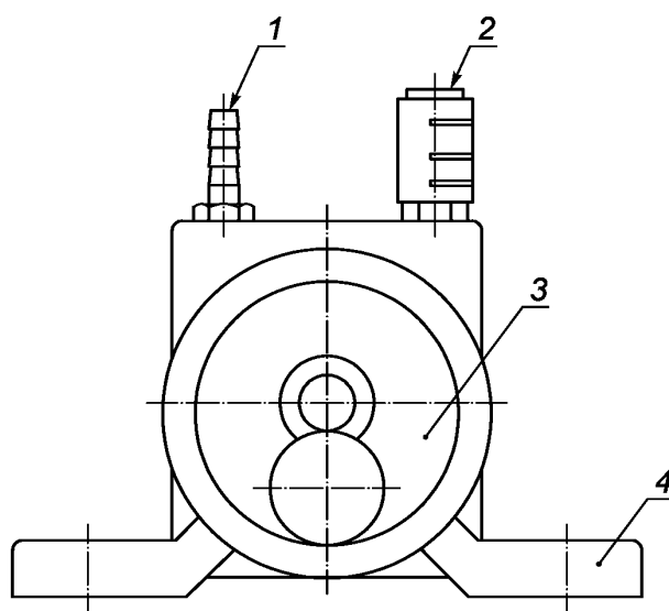
1 — шланг; 2 — глушитель; 3 — шарнир; 4 — станина
