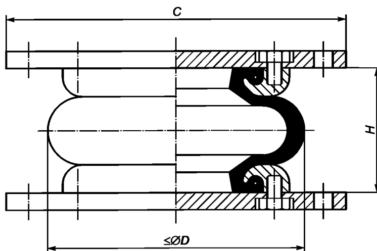
Рисунок В.4 — Основные размеры пневматической рессоры
